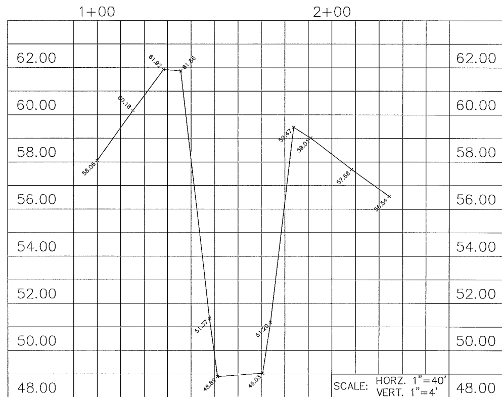
SECTION "FF-FF" STA. 12+32.3
