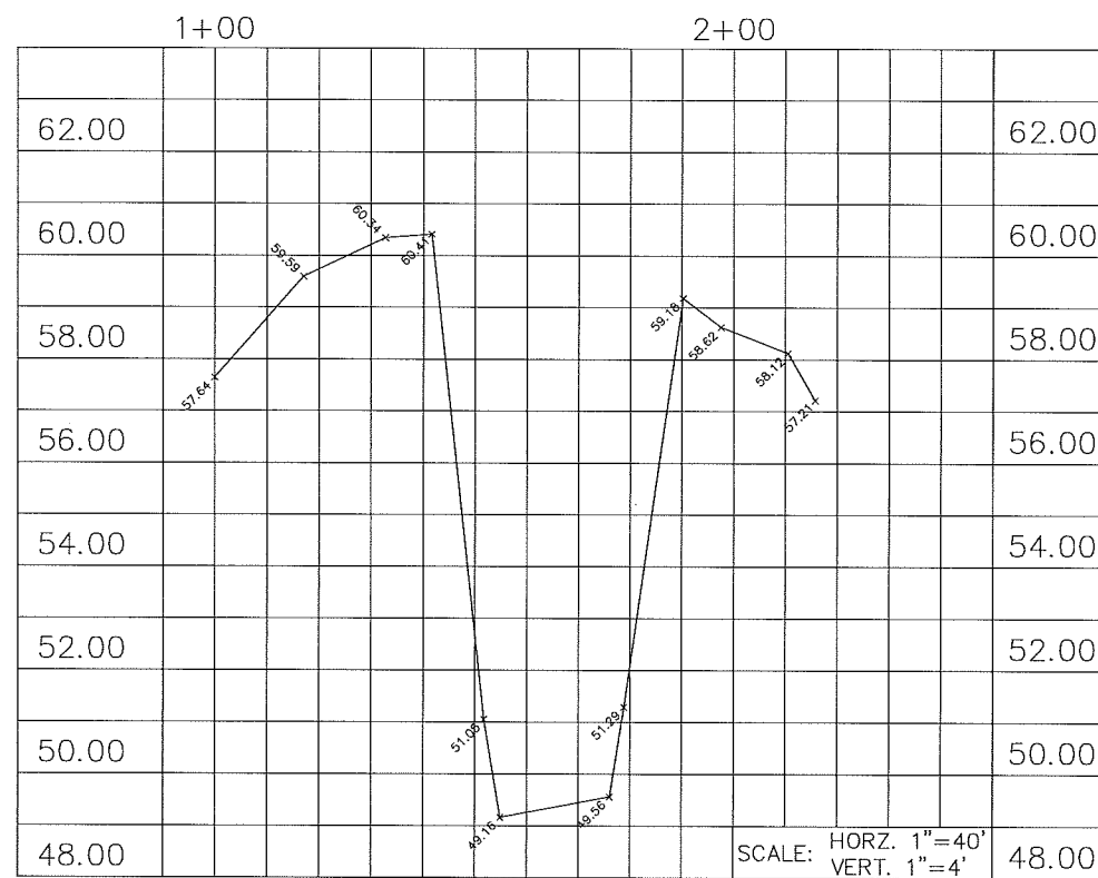
SECTION "DD-DD" STA. 15+17.5
