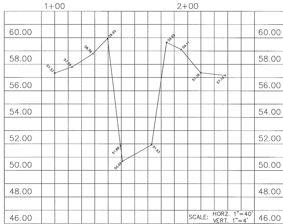
SECTION "J-J" STA. 36+83.4
