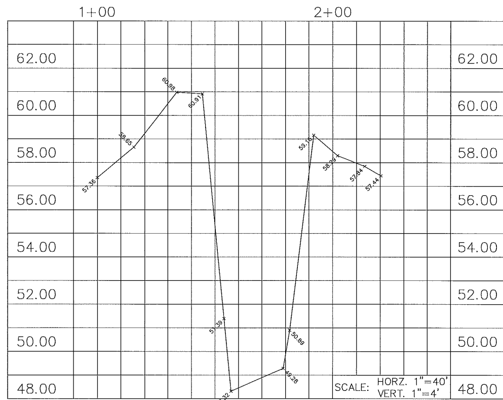
SECTION "CC-CC" STA. 16+10.5
