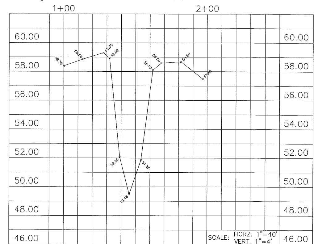
SECTION "AA-AA" STA. 7+95.3
