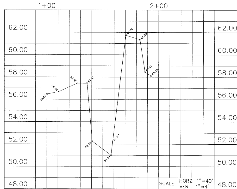
SECTION "N-N" STA. 76+71.6
