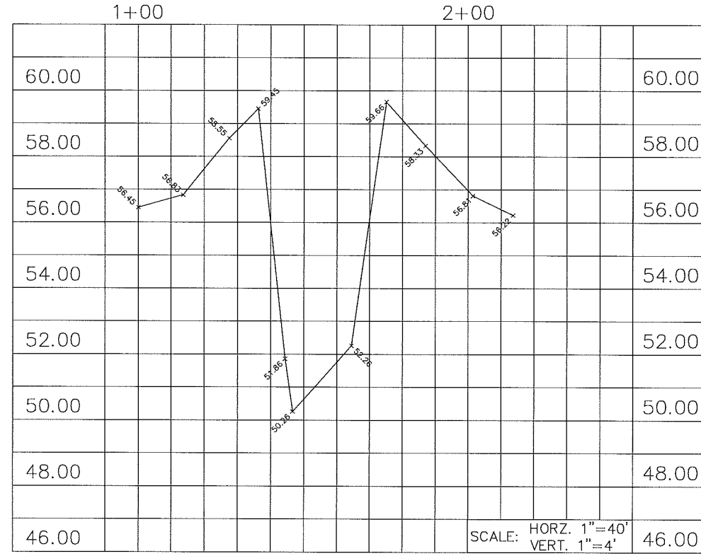
SECTION "K-K" STA. 65+72.5
