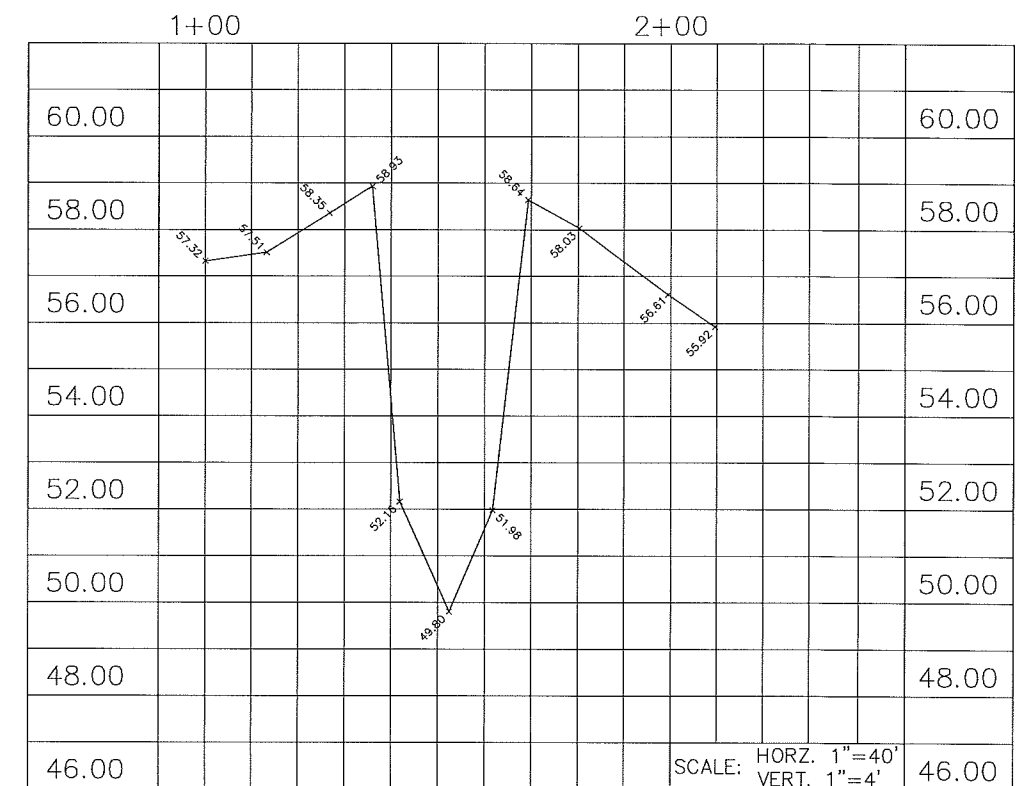
SECTION "L-L" STA. 66+40
