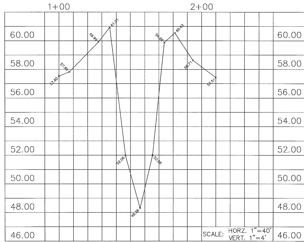
SECTION "M-M" STA. 67+65.9
