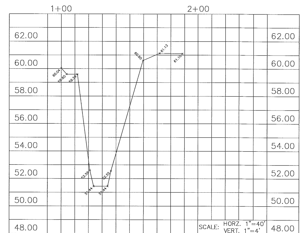
SECTION "X-X" STA. 134+06.6
