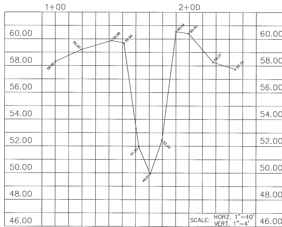
SECTION "Z-Z" STA. 7+05.1
