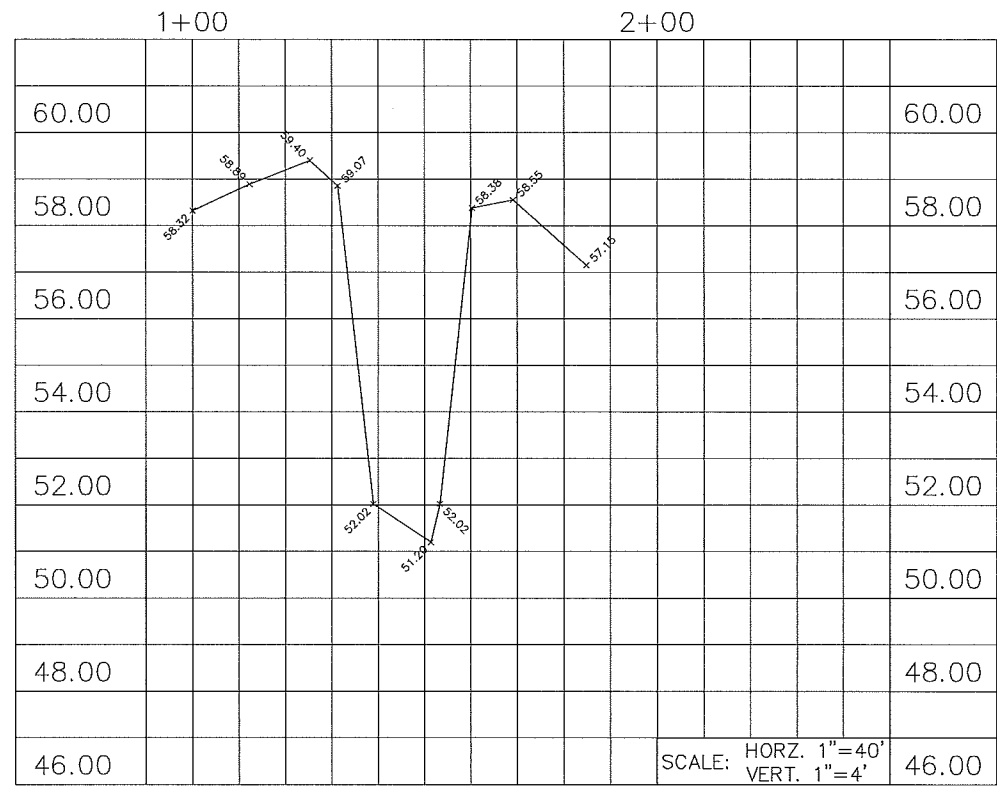
SECTION "BB-BB" STA. 8+80.7
