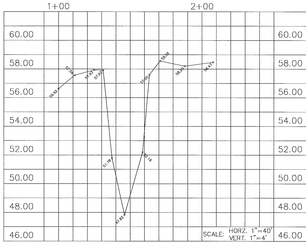
SECTION "P-P" STA. 78+58.7
