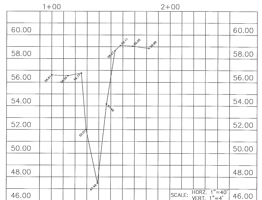
SECTION "O-O" STA. 77+43.8
