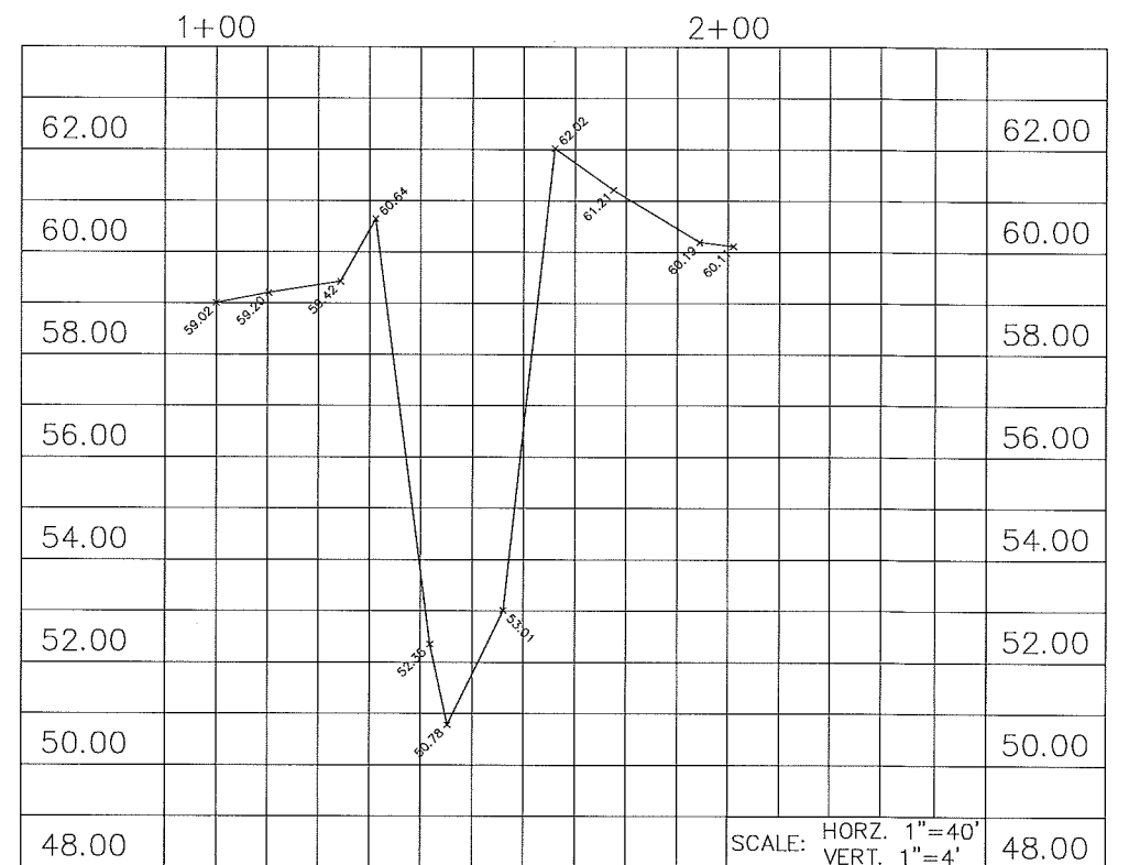
SECTION "R-R" STA. 119+05.9
