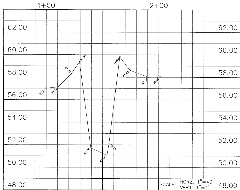
SECTION "Q-Q" STA. 79+37.1
