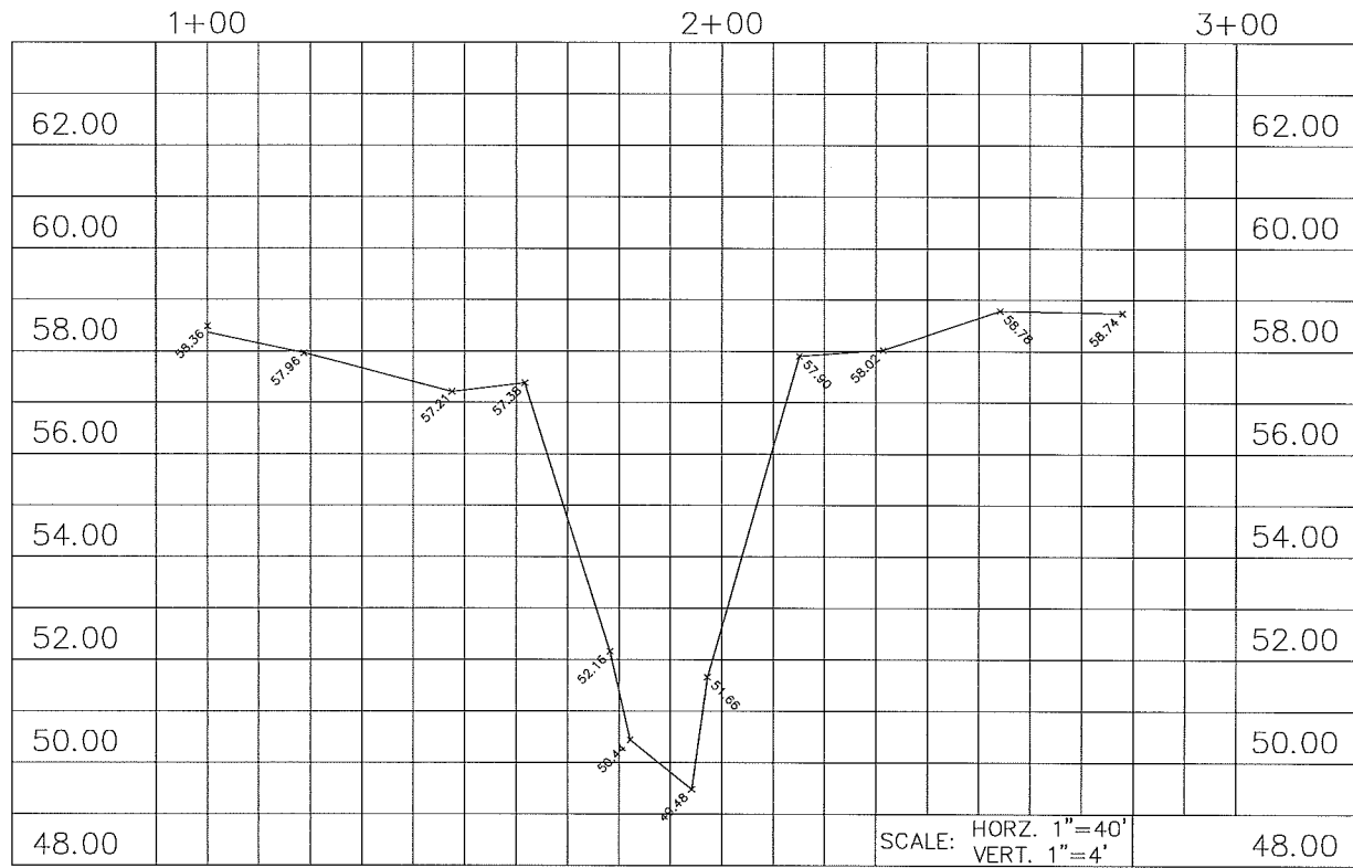
SECTION "C-C" STA. 15+02.6
